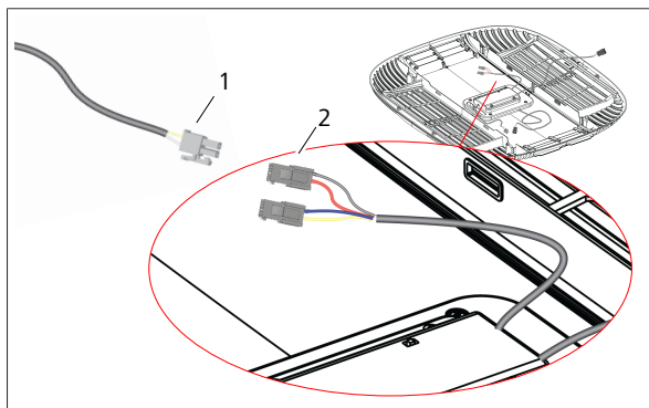
Afb. 24 Het CI-BUS-systeem aansluiten op de CI-BUS eenheid
