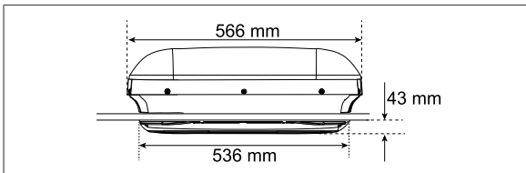
Afb. 8 Montage-afmetingen (vooraanzicht)
