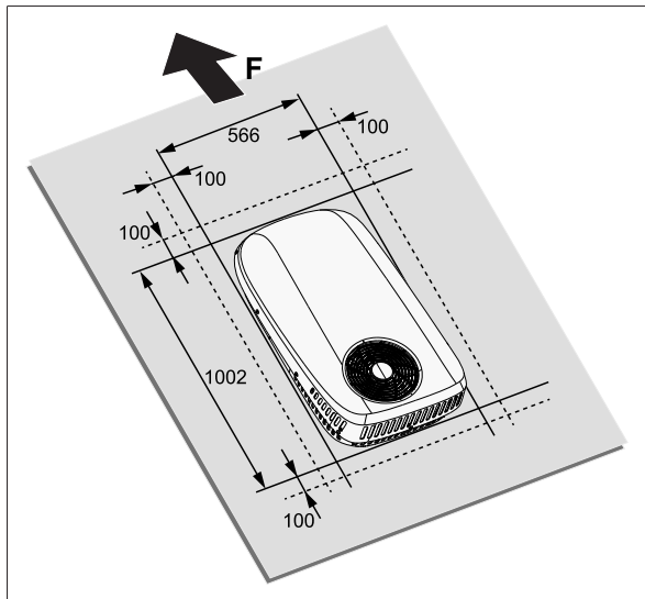
Afb. 5 Montagerichting van de buiteneenheid
