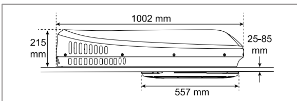
Afb. 7 Montage-afmetingen (zij-aanzicht)
