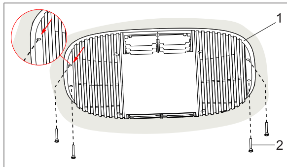
Afb. 29 De luchtverdeler vastmaken aan het dak
