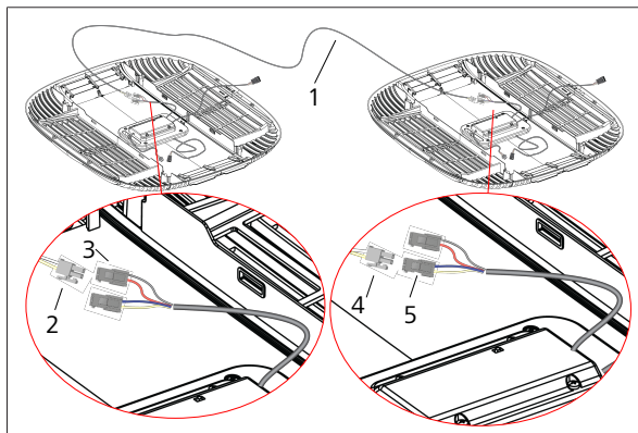
Afb. 26 Twee CI-BUS eenheden verbinden
