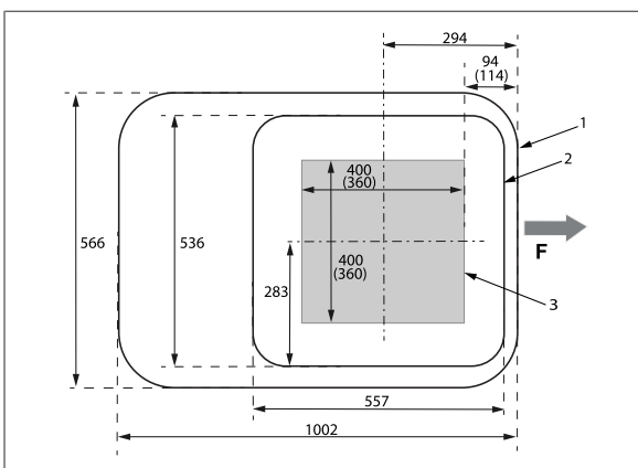
Afb. 6 Montage-afmetingen (boven-/onderaanzicht)
