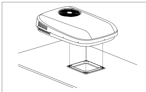
Afb. 18 De buiteneenheid plaatsen
