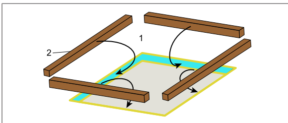
Afb. 9 Dakversterking
