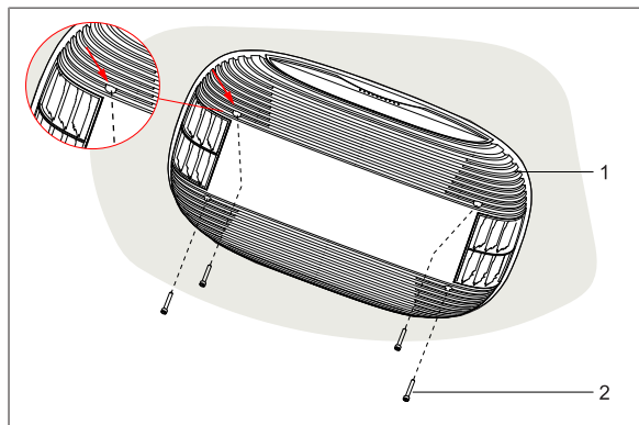
Afb. 28 De luchtverdeler vastmaken aan de bevestigingsbeugel
