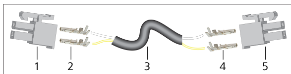
Afb. 14 Assemblage CI-BUS-interconnectiekabel tussen twee CI-BUS eenheden
