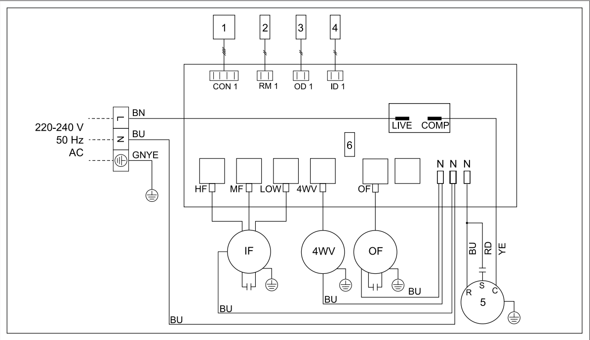
Afb. 56 Bedradingsschema
