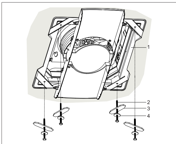
Afb. 20 De bouten monteren
