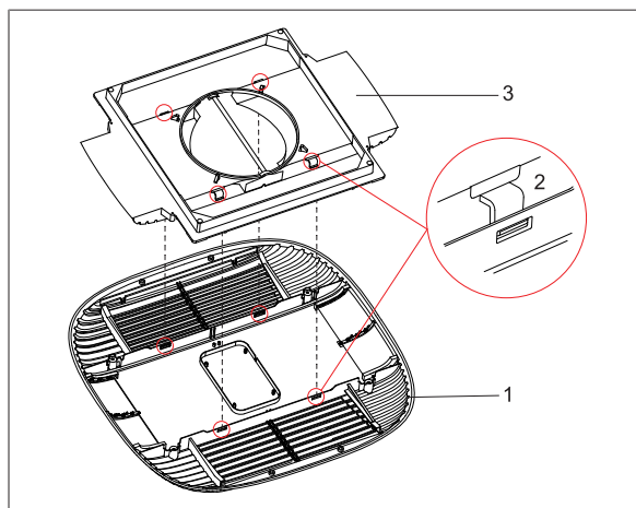
Afb. 27 De luchtverdeler bevestigen aan de bevestigingsbeugel
