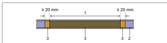
Afb. 10 Uitsnede met houten versterking
